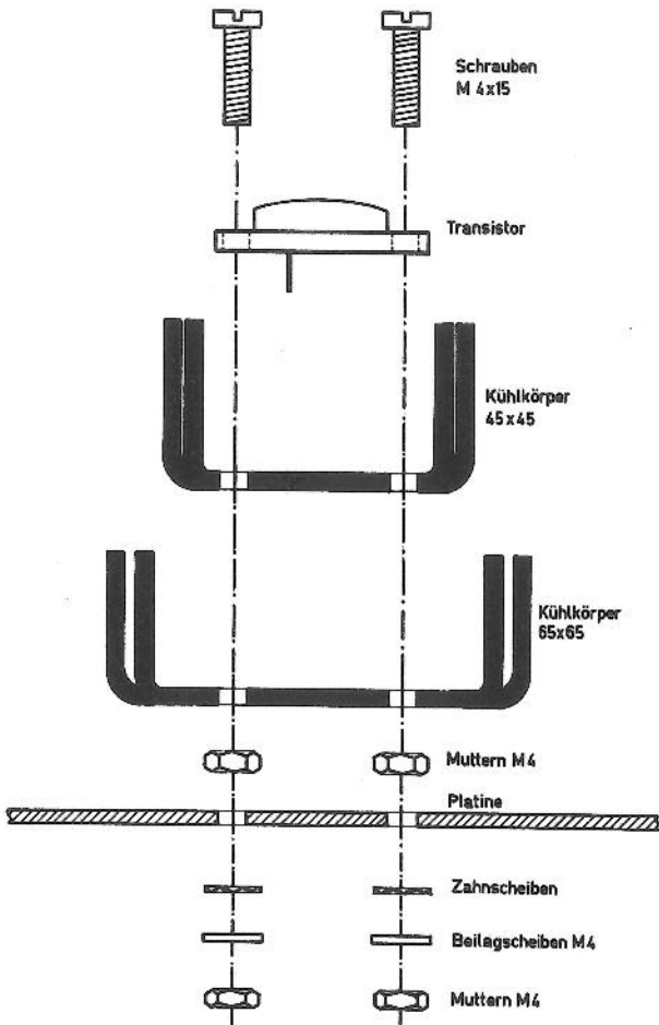
Abb. 11: Einbau der Transistoren Q 9 und Q 11
