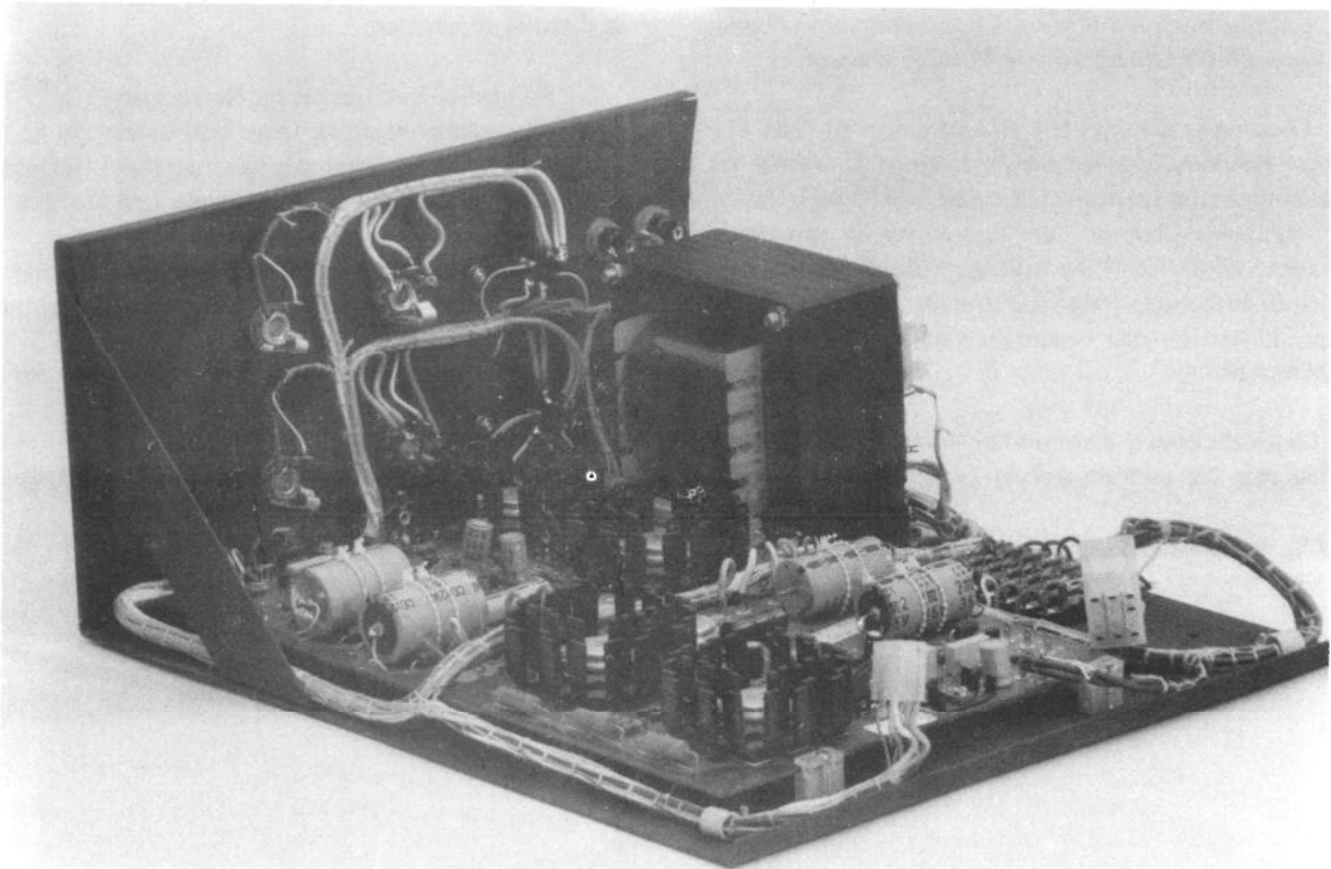
Abb. 2: Der zweikanalige Leistungseinschub LE 2
