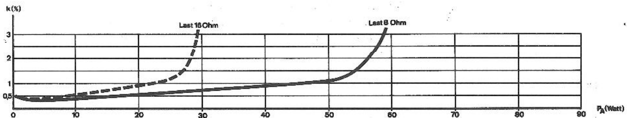
Abb. 6: Klirrfaktor der Endstufe bezogen auf eine Frequenz von 1000 Hz und eine Last von 8 bzw. 16 Ohm
