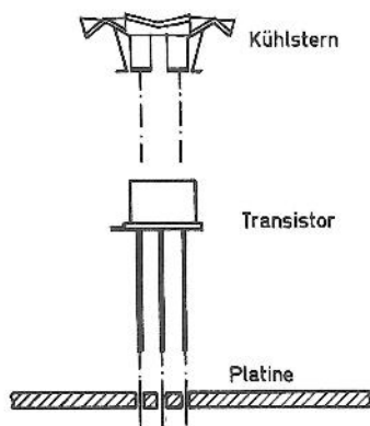
Abb. 9: Einbau des Transistors Q 5 mit Kühlstern
