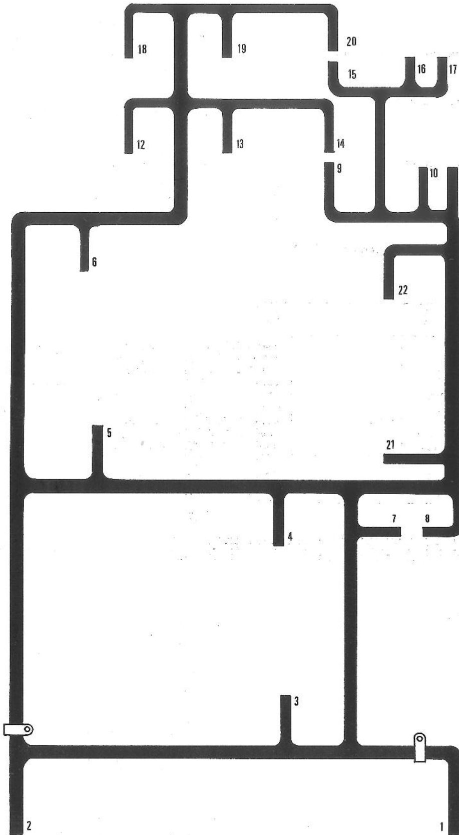
Abb. 19: Schematische Darstellung des Kabelbaumes LE 2
