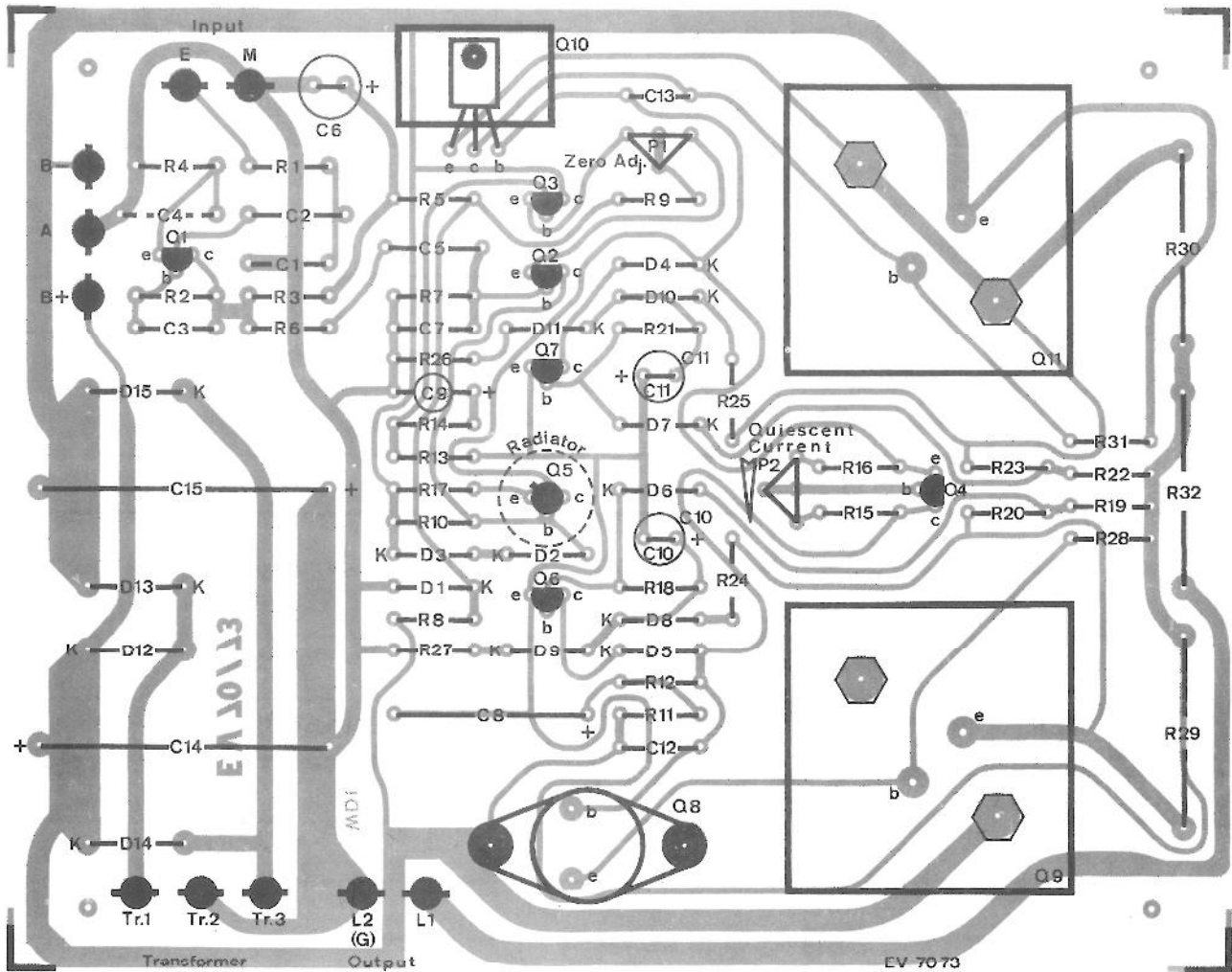
Abb. 8: Positionsdruck mit unterlegten Leiterbahnen der Platine EV 70
