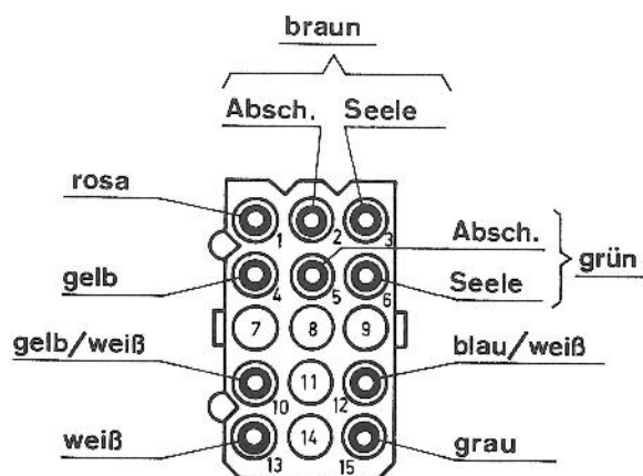
Abb. 20: "Kleine" Steckverbindung für LE 2
